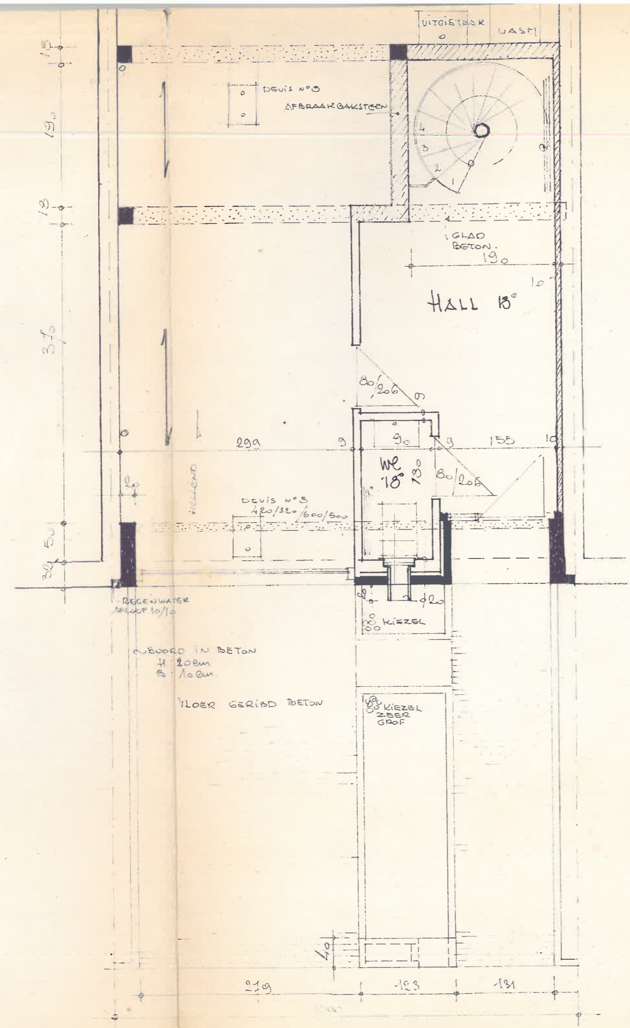
PLAN GELIJKVOER
